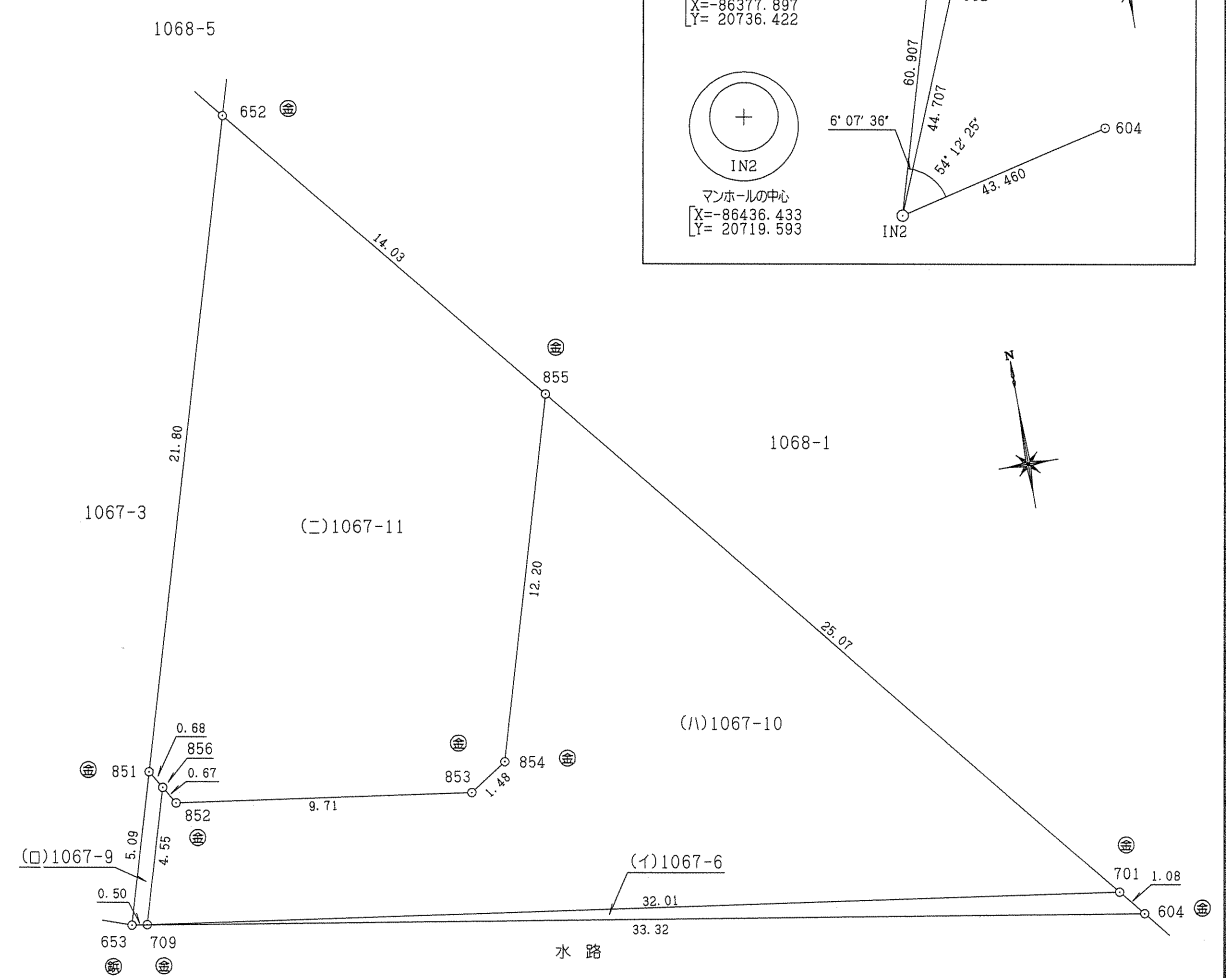
詳細図 Scale=1:50
